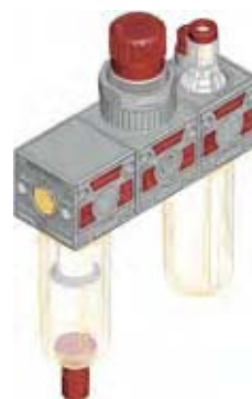
080-05 F + R + L - 0÷8 bar (sans manomètre)
