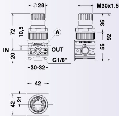
(A) TROUS DE FIXATION Ø 4,5
