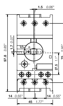
MS116 ≥ 20 A
