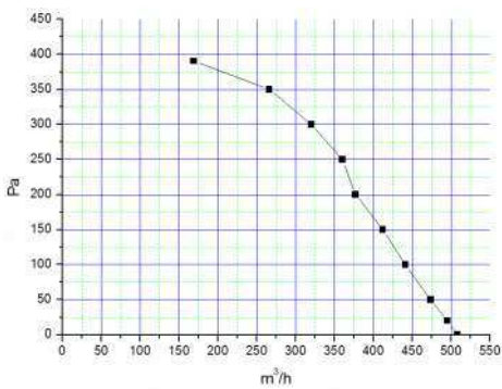
配蜗壳曲线
