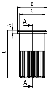
Gewindehülse Threaded Sleeve
