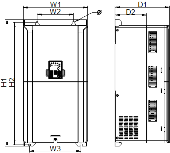
Montage mural des variateurs 3PH 380 V 45~75 kW
